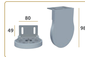
SOPORTE STANDARD
