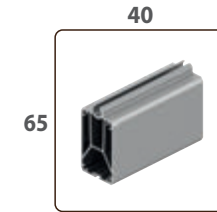
PERFIL CARGA
