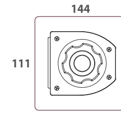
PERFIL COFRE
