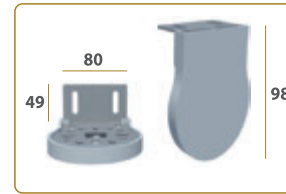
SOPORTE STANDARD
