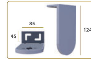
SOPORTE LARGO
