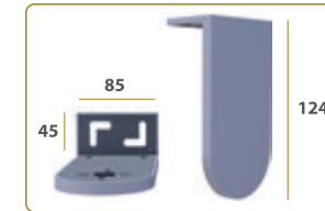
SOPORTE LARGO
