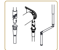
MANIVELA ARTICULADA
