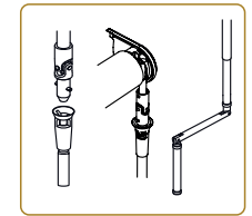
MANIVELA ARTICULADA
