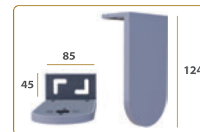
SOPORTE LARGO
