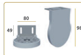
SOPORTE STANDARD
