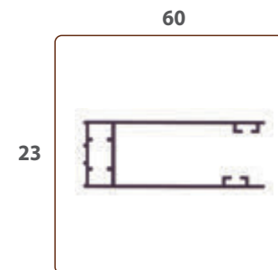
PERFIL GUÍA
