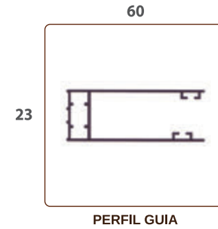
PERFIL GUIA
