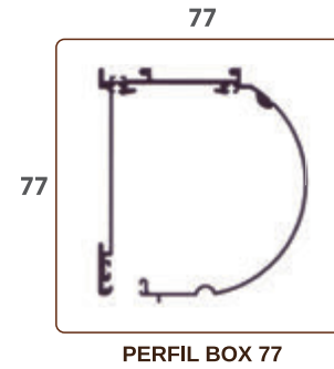
PERFIL BOX 77
